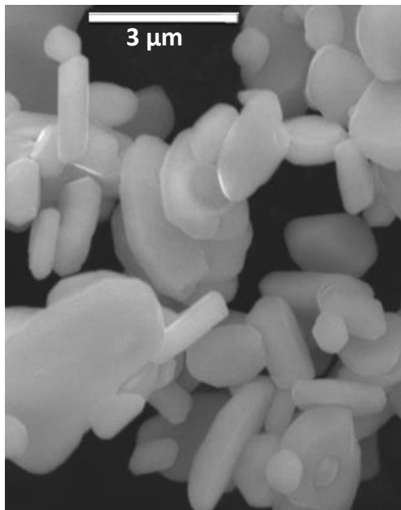
NiTiO 3 calcinado a 850°C
