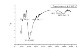
Fig.3 Espectroscopia IR del \beta -espodumeno
