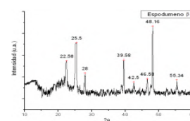
Fig.2. Difractograma de \beta -espodumeno
