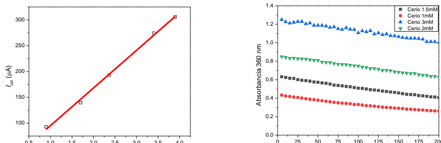
Fig. 1 Variación de I_{cat} vs [1] (izq) y de la absorbancia a 360 nm vs [Ce(IV)] (der.) a pH = 1 (ácido trifílico 0,1 M).
